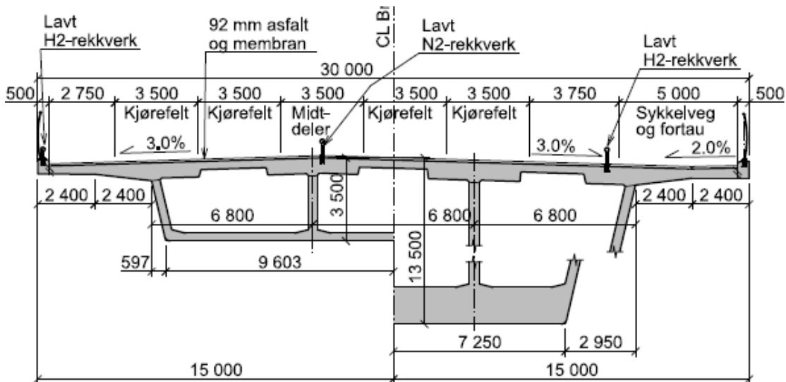
TVERRSNITT FFB
